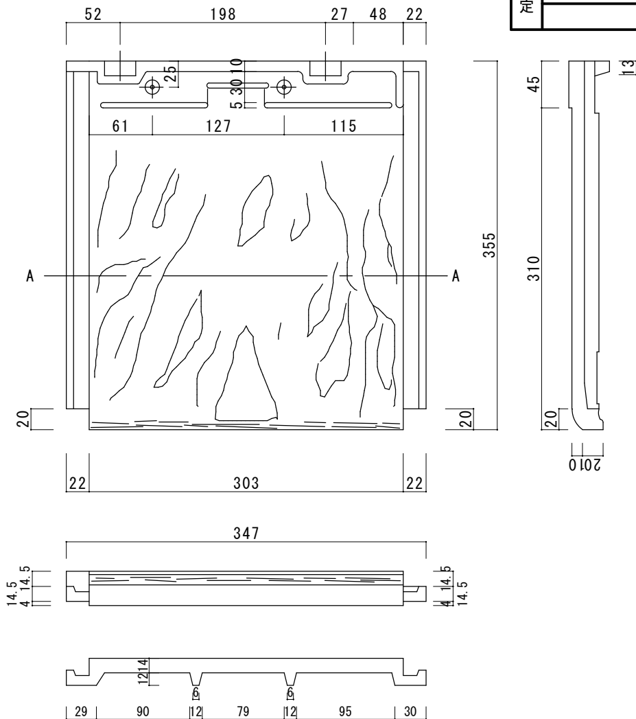
A-A 断面図
