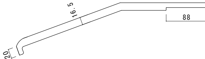
A-A 断面図
