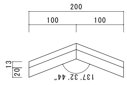
A-A 断面図
