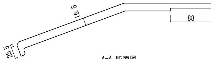
A-A 断面図
