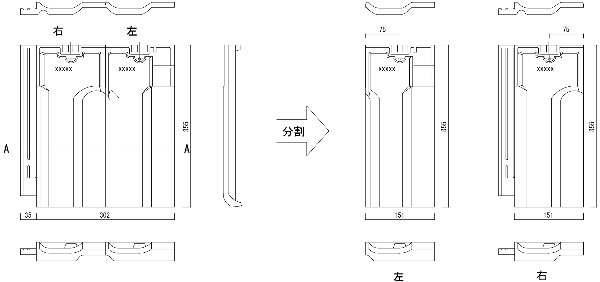
A-A 断面図
