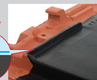
高い水返し
